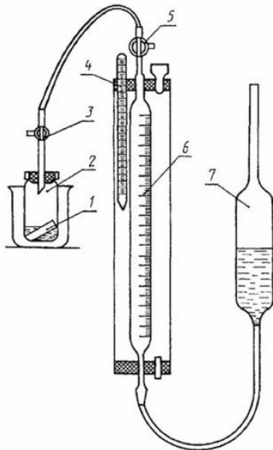
Рисунок 1. 1 — стеклянная пробирка по ГОСТ 25336; 2- сосуд типа СЦ-0,5 по ГОСТ 25336; 3, 5 — краны соединительные по ГОСТ 7995; 4 — термометр по ГОСТ 28498; 6 — бюретка типа 3-2-100-0,2 по ГОСТ 29252-91; 7 — уравнивательная склянка по ГОСТ 25336
